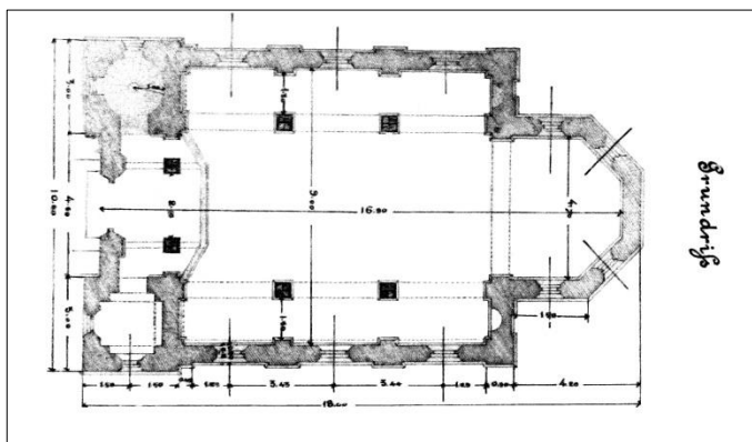
Типски пројекат за гркокатоличку цркву, 1884, основа
