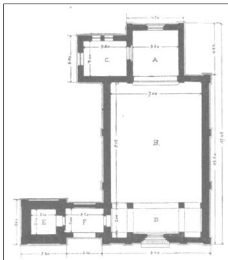
Slika 3. Osnova izvedenog Vancaševog projekta crkve. A – oltarski prostor, B – naos, C – sakristija, D – narteks, E – zvonik, F – galerija
