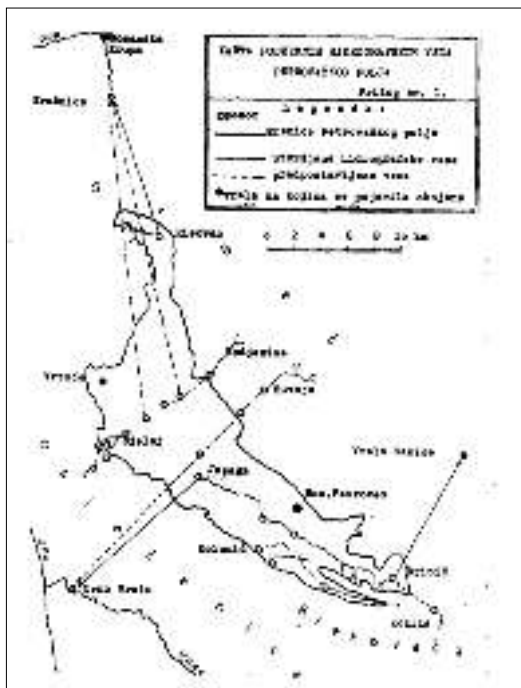
Слика 2. Вођеница на карти подземних хидрографских веза Петровачког поља 3
