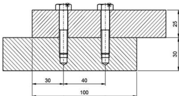
Slika 8 - Dve zavrtnjske veze sa dve nalegle ploče [14]
