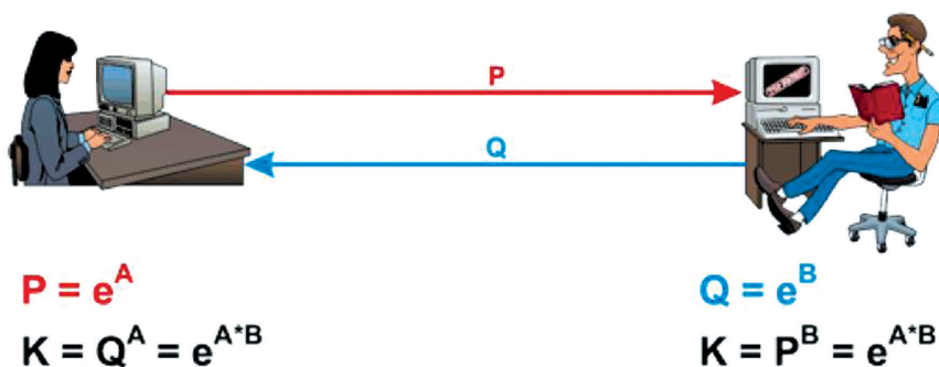
Слика 3. Дифи-Хелманов протокол
