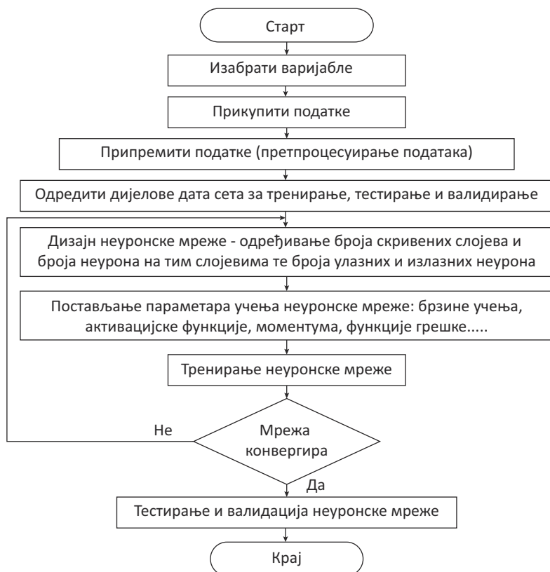
Слика 3. Кораци алгоритма дизајна умјетне неуронске мреже. Извор: Аутори
