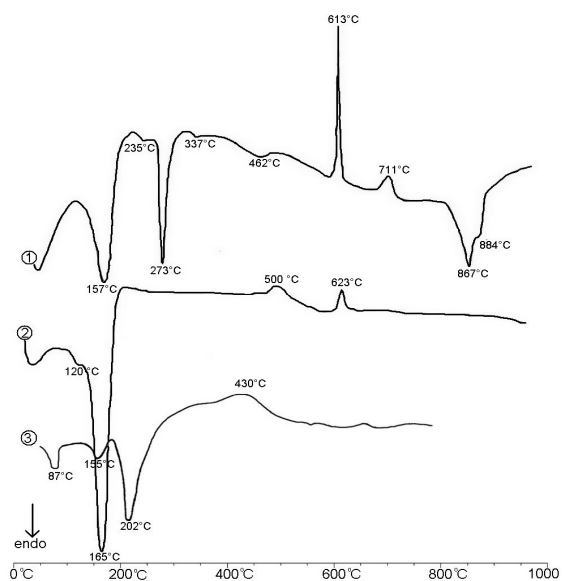
Figure 3 DTA diagrams: 1) vivianite; 2) ludlamite; 3) vauxite
