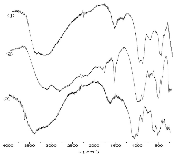
Figure 4 IR spectra: 1) vivianite; 2) ludlamite; 3) vauxite
