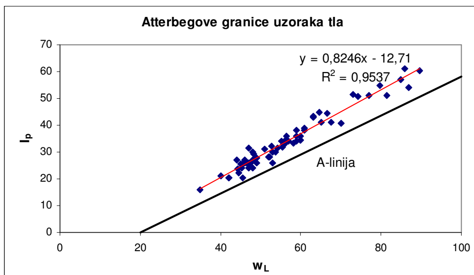
Slika 1 Korelacija između granice tečenja i indeksa plastičnosti
