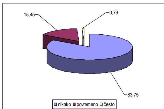
Grafikon 3.1.1.1: Distribucija rezultata procjene raširenosti oblika asocijalnog ponašanja učenika
